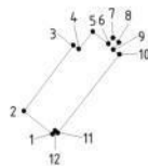
5.20. Чертеж границ земельного участка с кадастровым номером 70:22:0010103:з/у286 М 1:1000
