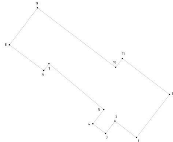
5.17. Чертеж границ земельного участка с кадастровым номером 70:22:0010103:з/у277 М 1:1000
