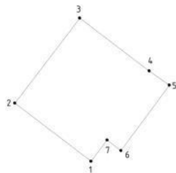
5.18. Чертеж границ земельного участка с кадастровым номером 70:22:0010103:з/у278 М 1:1000
