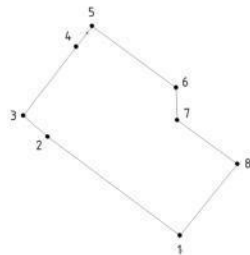
5.14. Чертеж границ земельного участка с кадастровым номером 70:22:0010103:з/у273 М 1:1000
