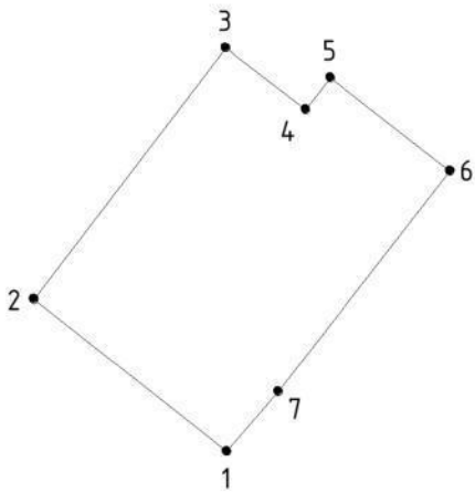
5.23. Чертеж границ земельного участка с кадастровым номером 70:22:0010103:з/у305 М 1:1000
