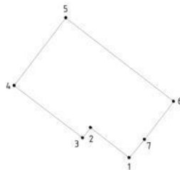
5.15. Чертеж границ земельного участка с кадастровым номером 70:22:0010103:з/у275 М 1:1000
