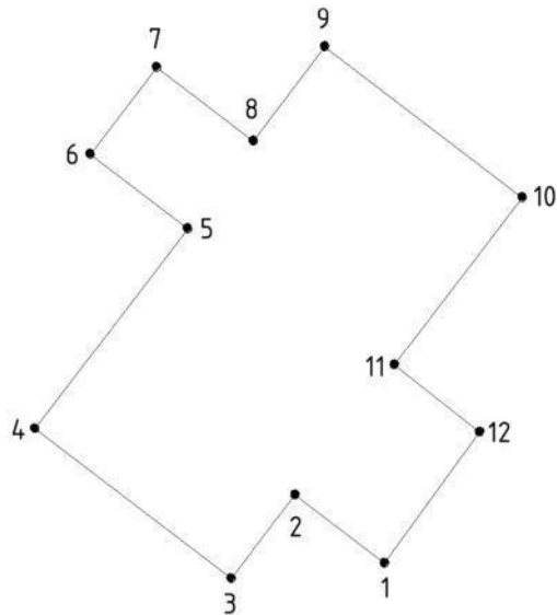
5.29. Чертеж границ земельного участка с кадастровым номером 70:22:0010103:з/у4119 М 1:1000
