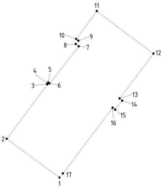
5.6. Чертеж границ земельного участка с кадастровым номером 70:22:0010103:55 М 1:1000
