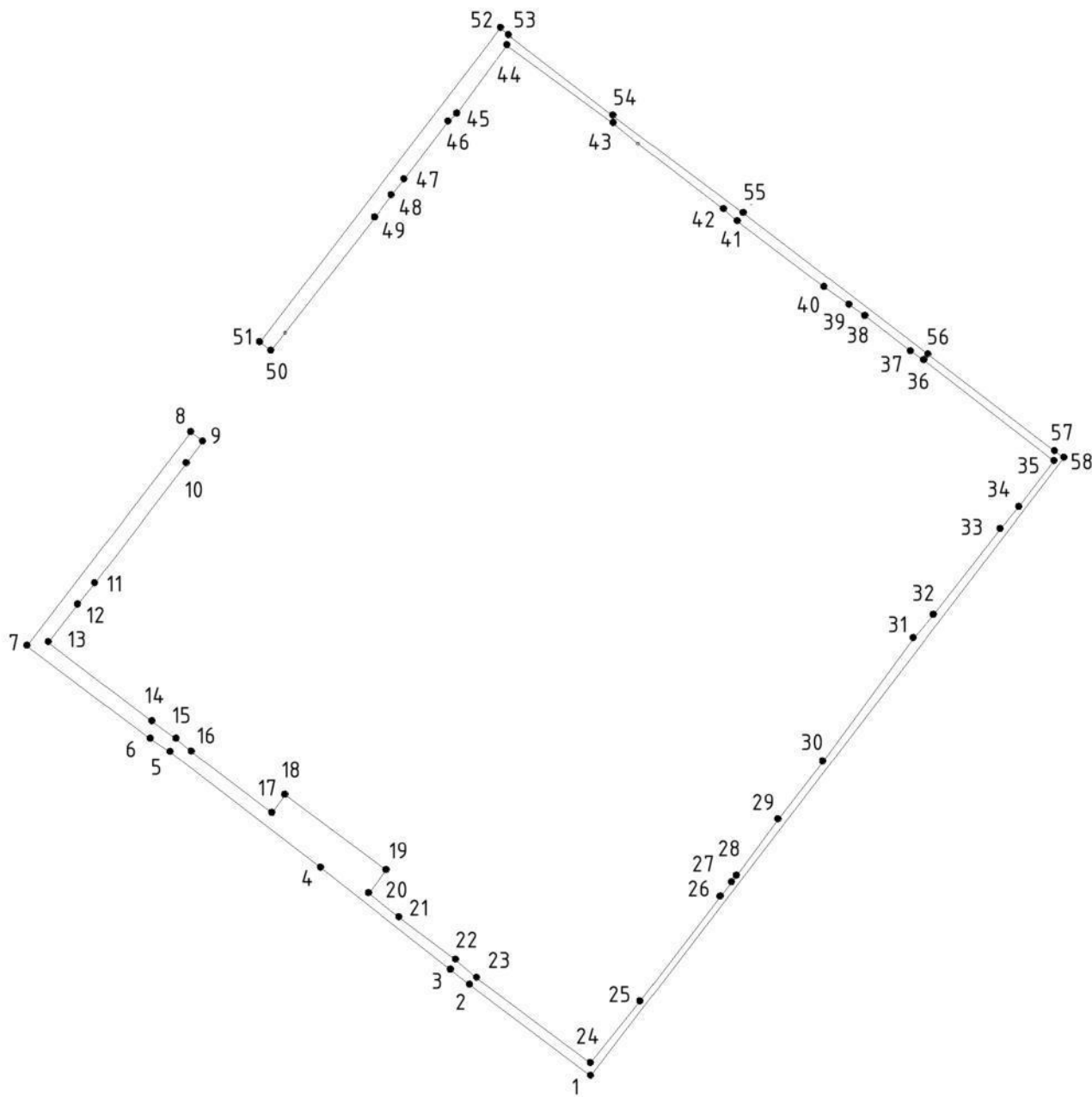
5.2. Чертеж границ земельного участка с кадастровым номером 70:22:0010103:з/у01 М 1:2000
