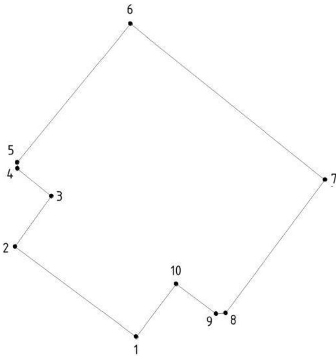
5.9. Чертеж границ земельного участка с кадастровым номером 70:22:0010103:з/у114 М 1:1000
