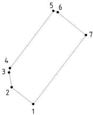
5.10. Чертеж границ земельного участка с кадастровым номером 70:22:0010103:з/у130 М 1:1000
